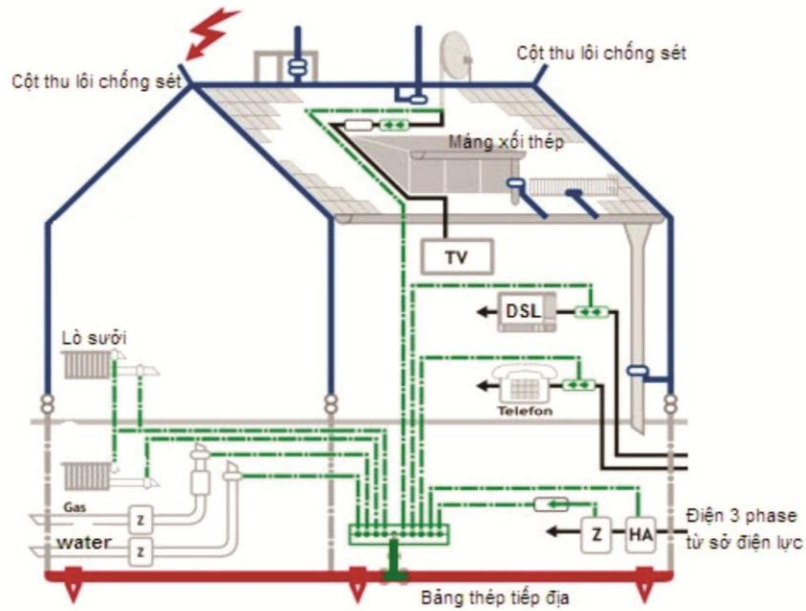
Sơ đồ tòa nhà lắp đặt hệ thống chống sét đánh thẳng và hệ thống chống sét đánh lan truyền
