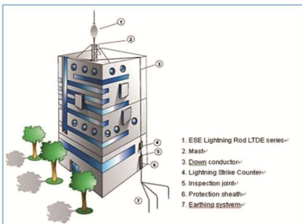
Hệ thống chống sét đánh thẳng
